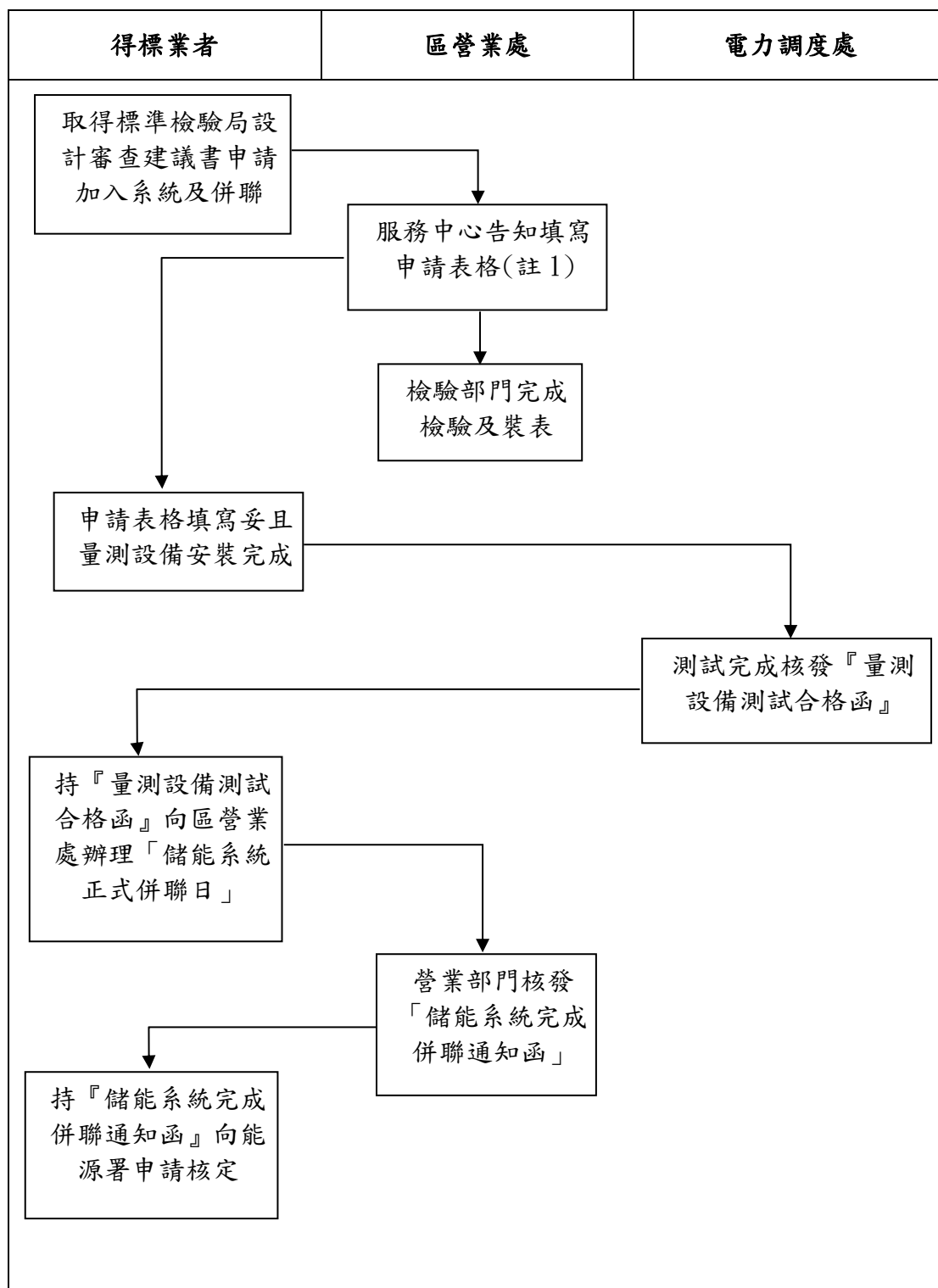
附圖 6 儲能系統結合太陽光電發電設備之儲能系統加入電力系統流程
