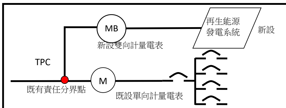
圖1-1 併聯至既有責任分界點之表位示意圖
