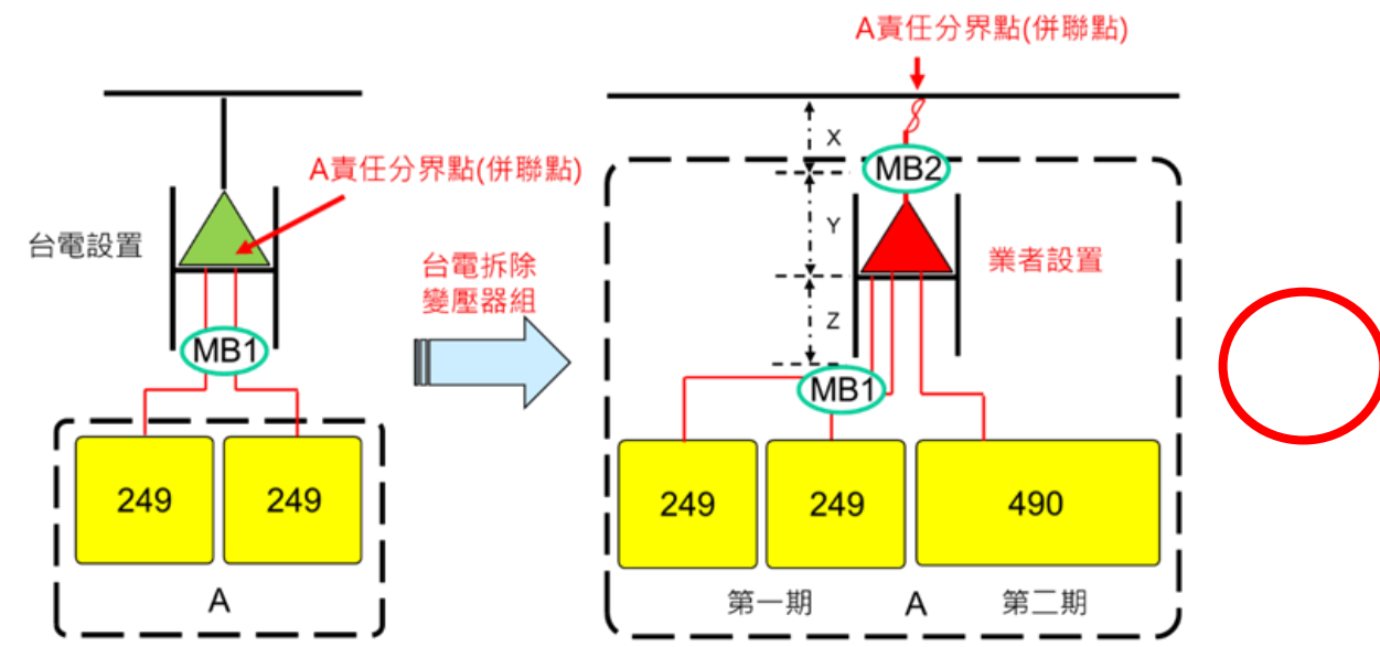
圖6. 同一場址同一(不同)設置者申請2案合併計算容量達500kW 以上且共用一併聯點引接線
