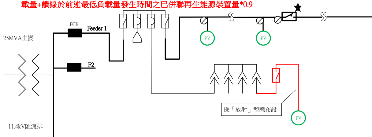
圖 3 近太陽光電案場（或合適地點）裝設「地下二路自動線路開關」
