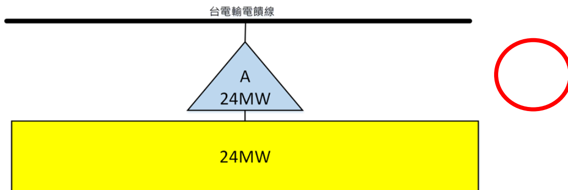
圖 2. 整合 1 案申設併接特高壓系統接線圖
