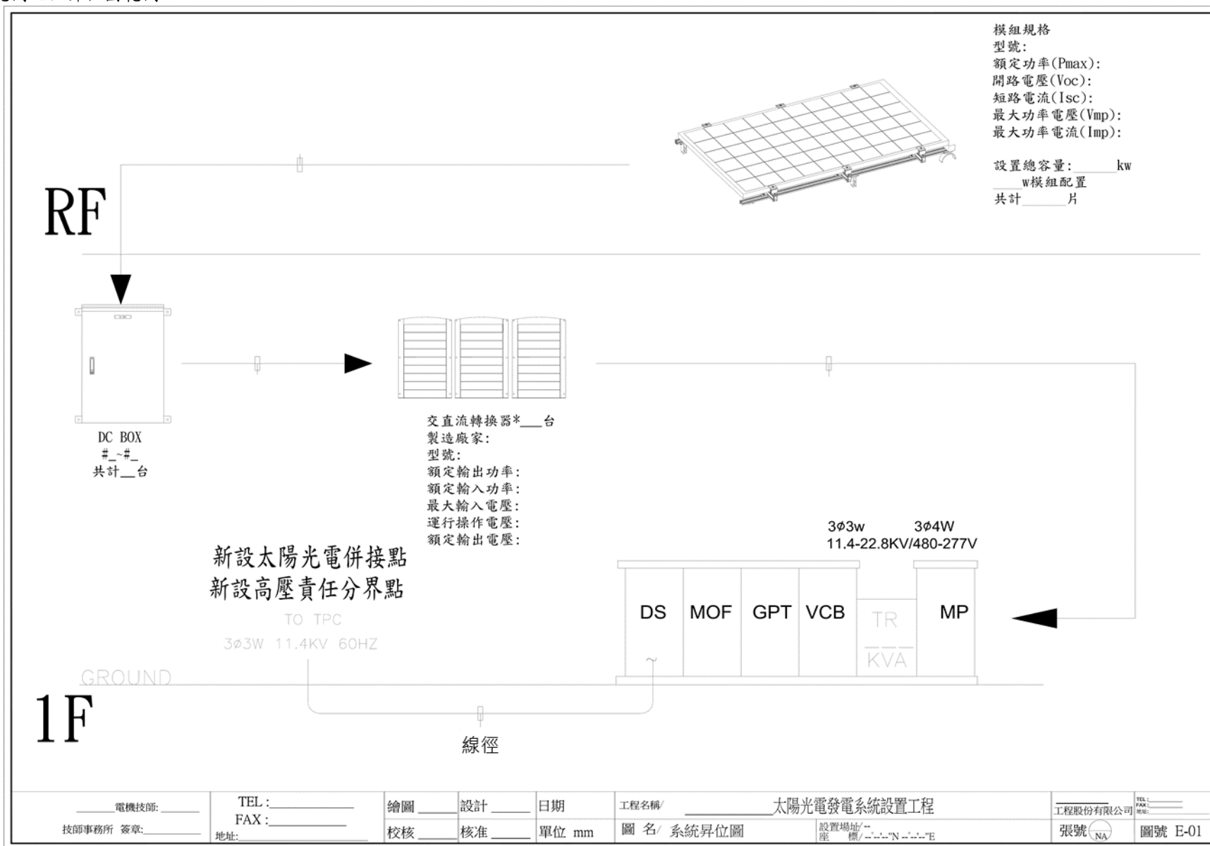
範例 10 昇位圖範例
