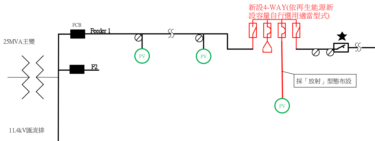
圖 2 近太陽光電案場（或合適地點）裝設「地下四路自動線路開關」
