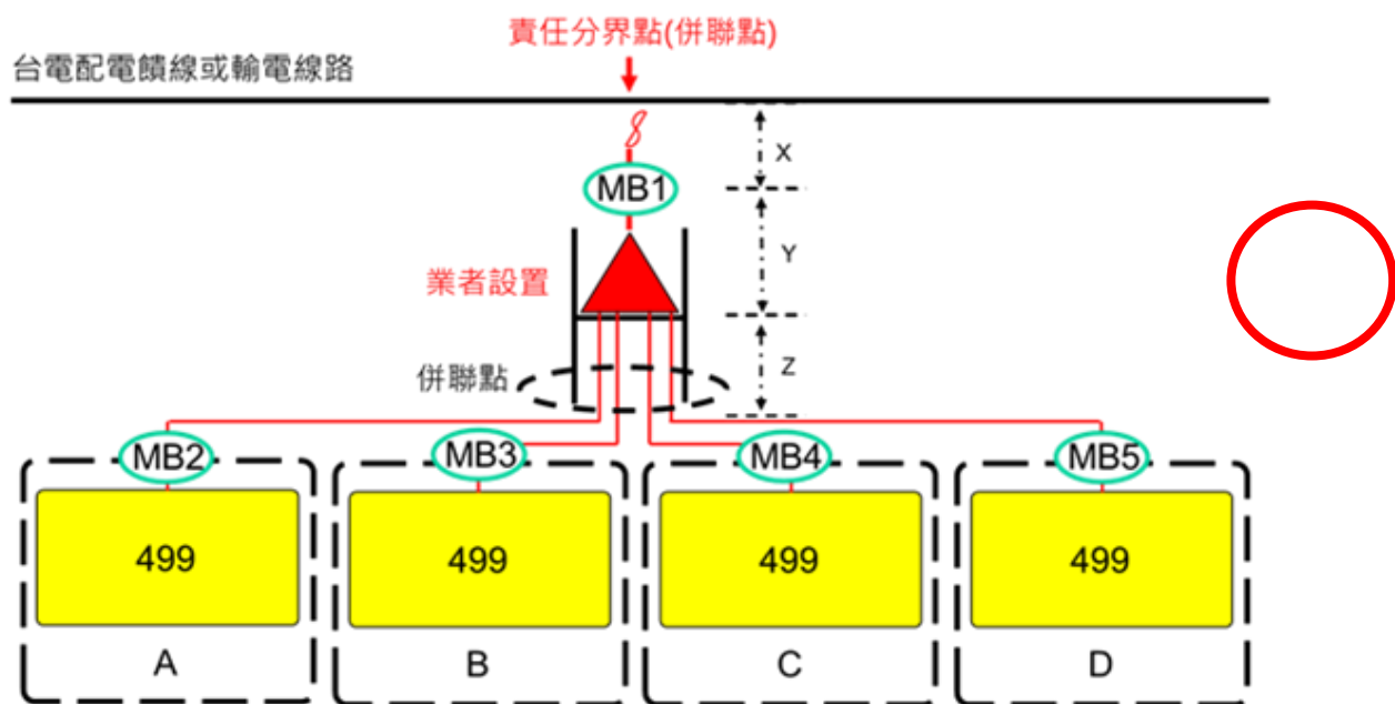
圖 3. 同一場址不同設置者申請多案共用(同)升壓站(變壓器)與引接線路
