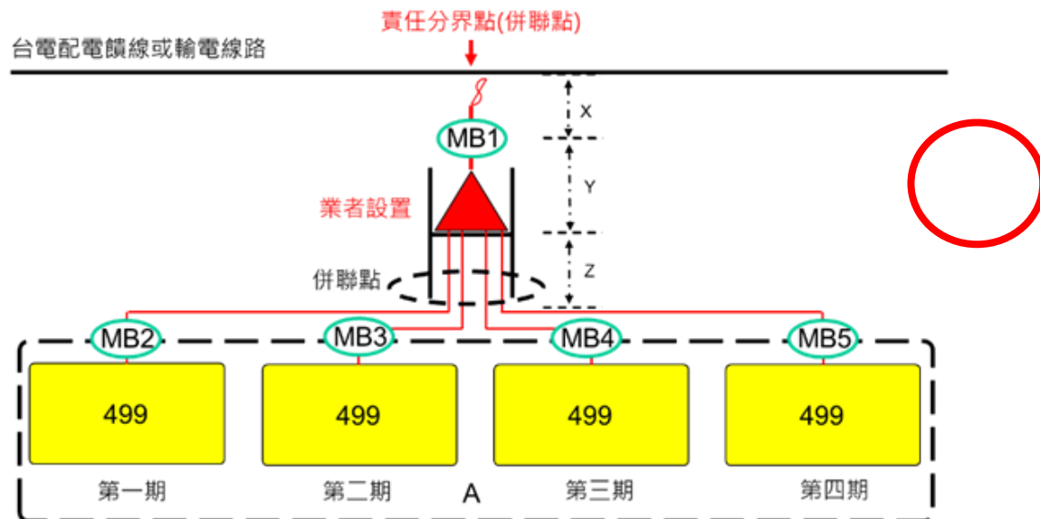
圖 5. 同一場址同一設置者申請多案共用(同)升壓站(變壓器)與引接線路且各案躉購費率不同引接線路圖
