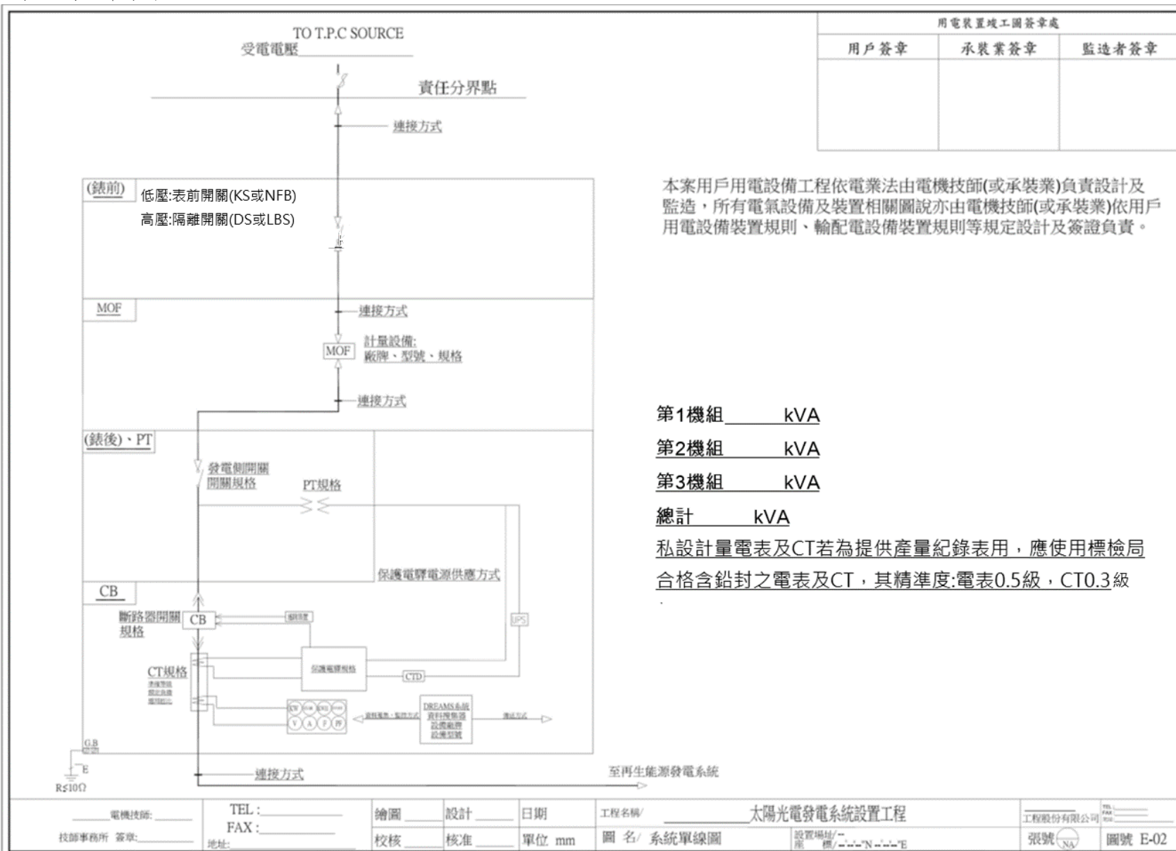
範例 11 系統單線圖
