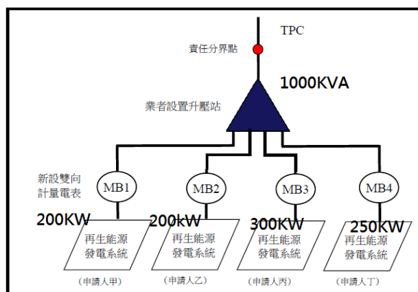
圖 4-4 不同人(同時)申請多案共用升壓站之表位示意圖
