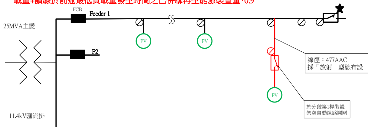
圖 4 近太陽光電案場（或合適地點）裝設「架空自動線路開關」
