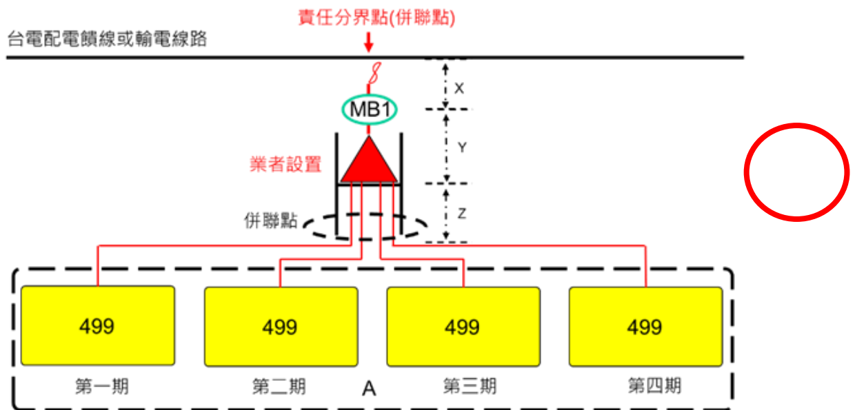
圖 4. 同一場址同一設置者申請多案共用(同)升壓站(變壓器)與引接線路且各案躉購費率相同引接線路圖
